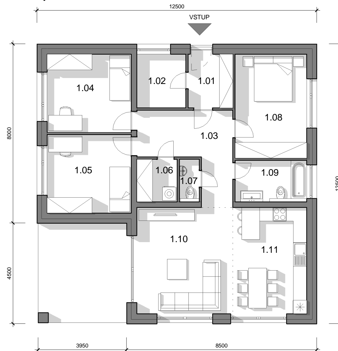
Pôdorys domu
